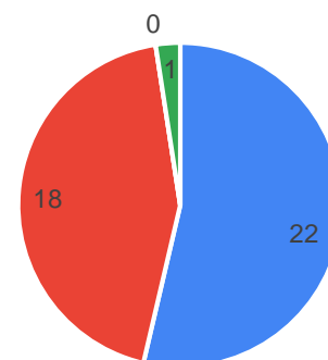
アンケート参加者(性別)
